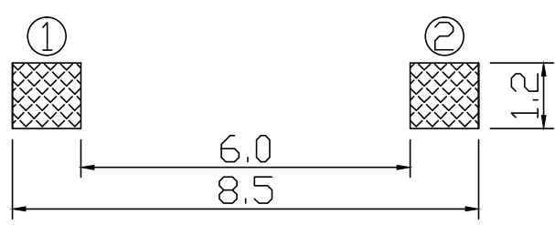
Reference P.C.B Layout
