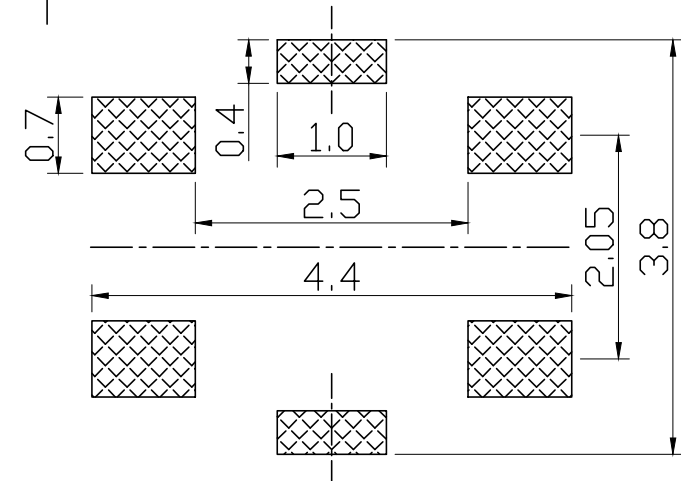
P.C.B Layout
