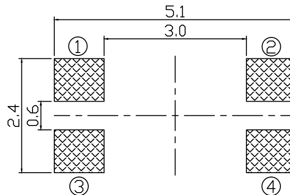
P.C.B Layout
