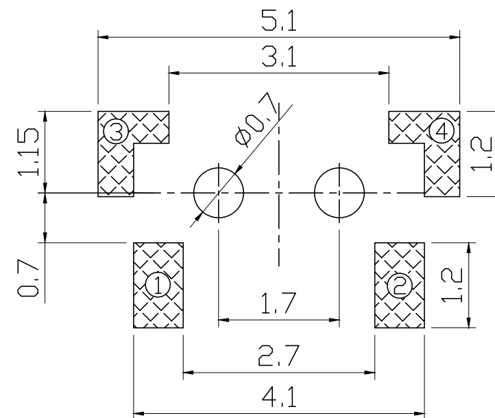
P.C.B. Layout
